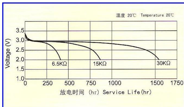
电阻容量曲线 Load-capacity
